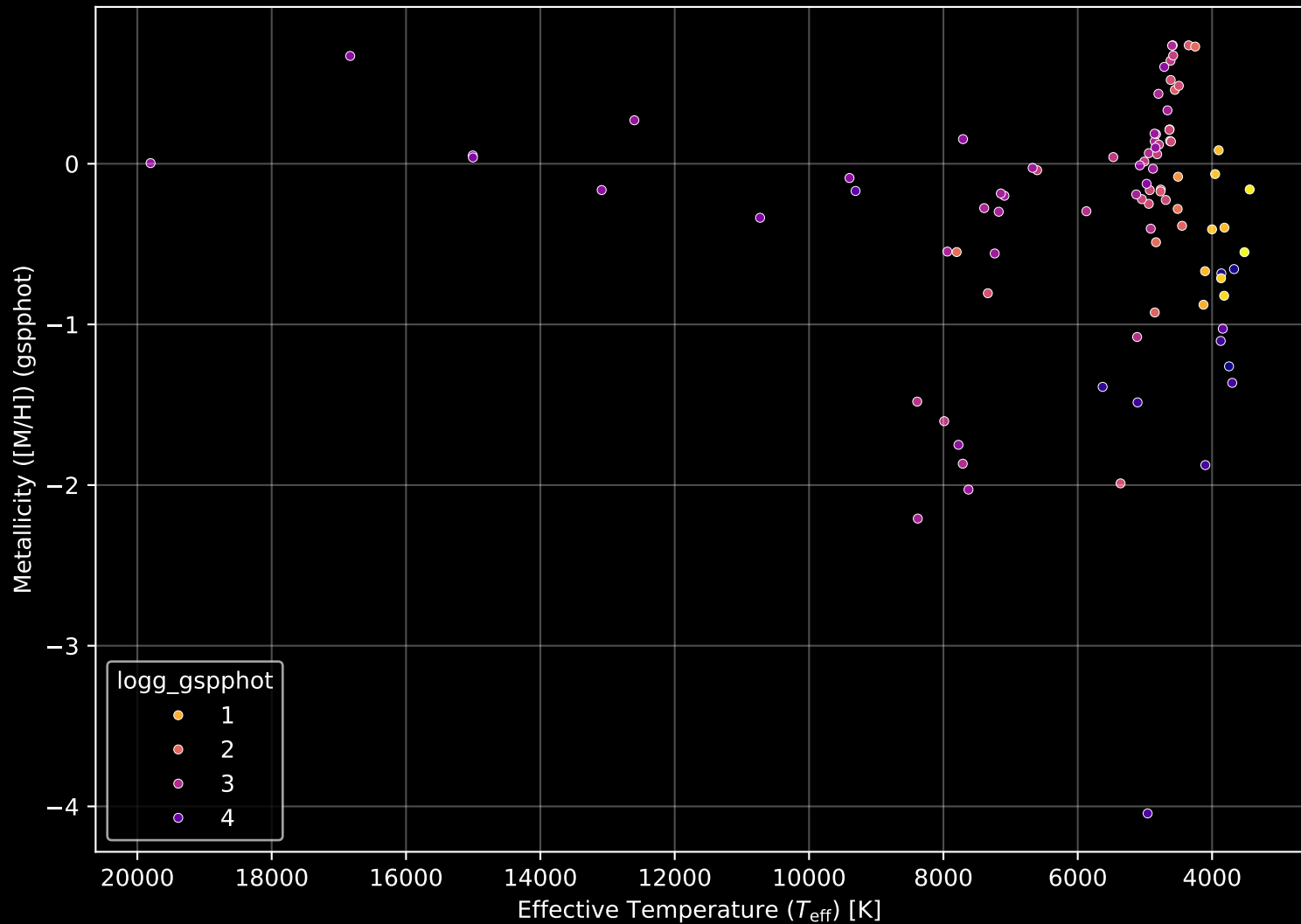
APOGEE DR17 Field: [013+00] Stellar Population Parameters (n= 90)
